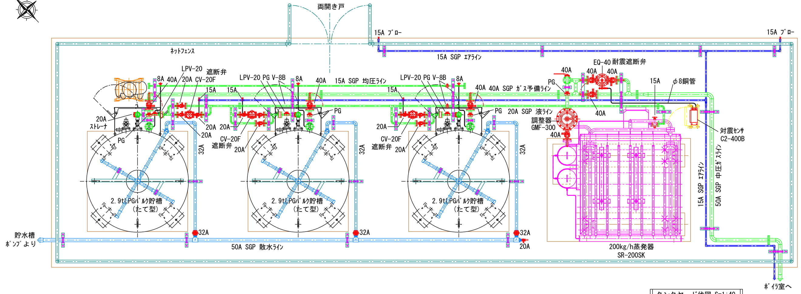
タンクヤード伏図 S=1:40
