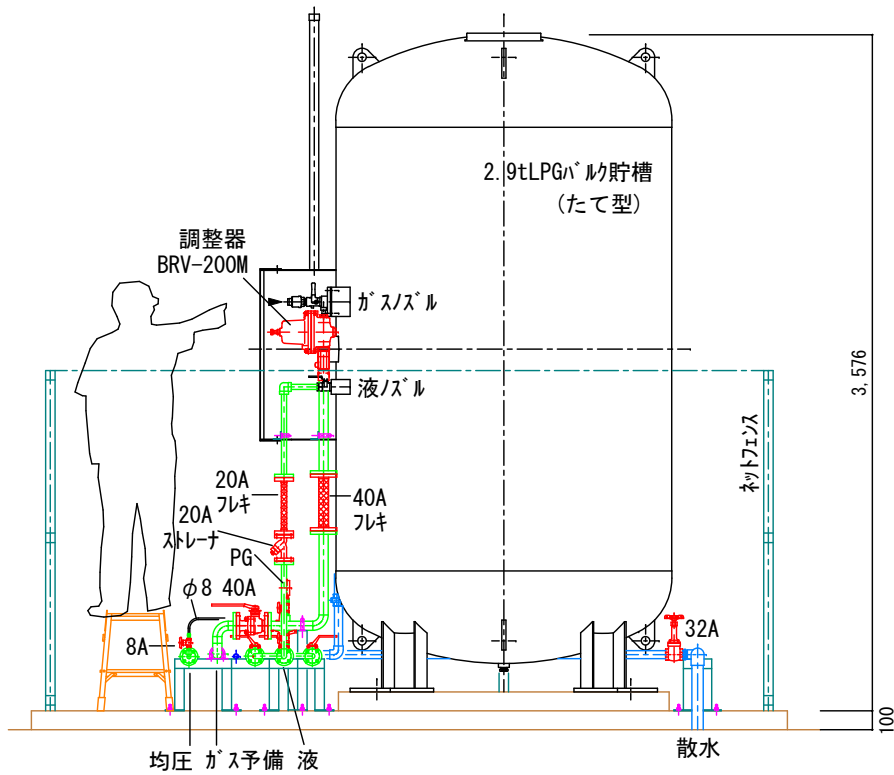
貯槽取出部詳細 S=1:40
