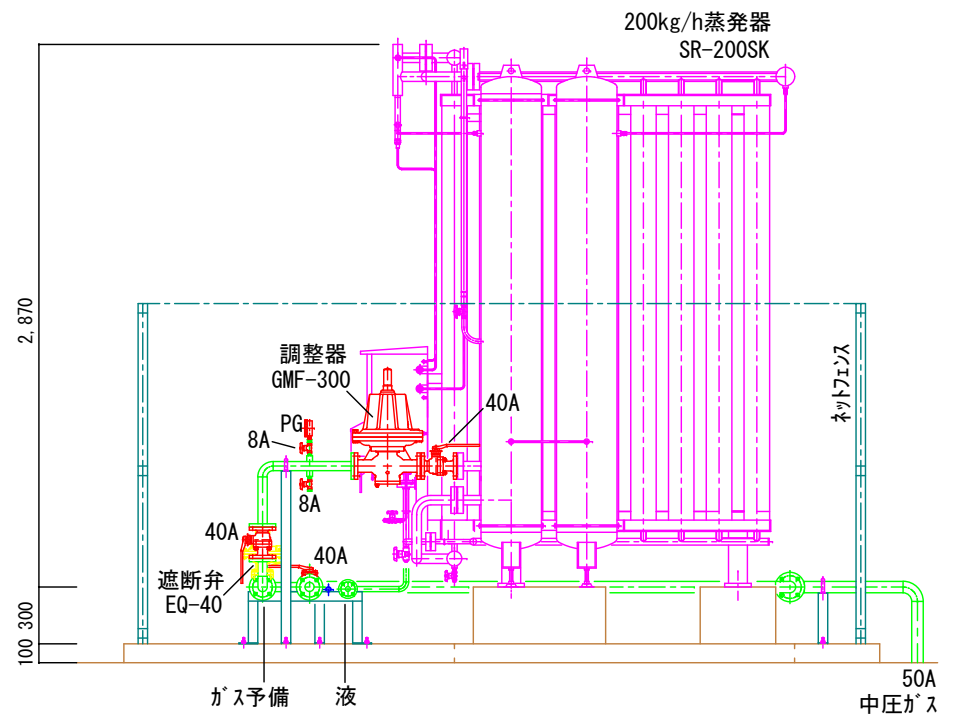
蒸発器取出部詳細 S=1:40
